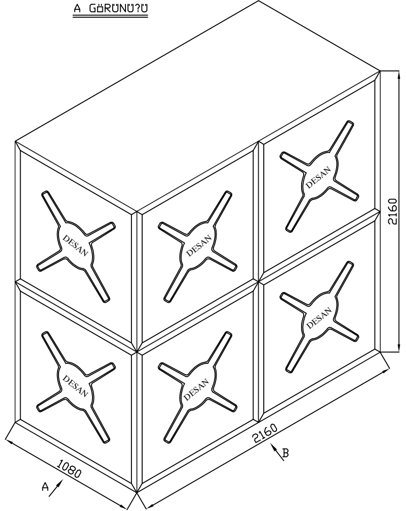
GENEL GÖRÜNÜŞÜ
