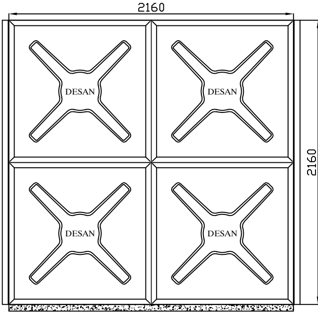
B GÖRÜNÜŞÜ
