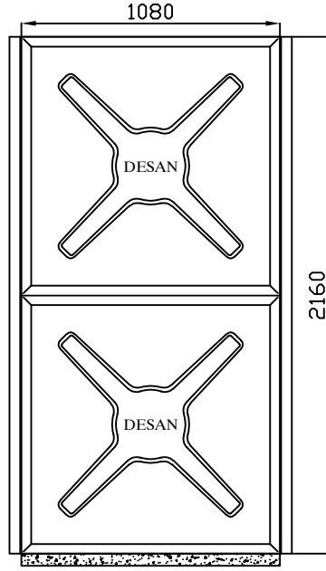
A GÖRÜNÜŞÜ
