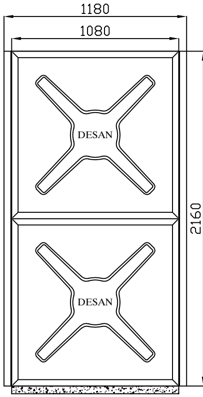
B GÖRÜNÜŞÜ
