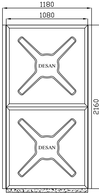
A GÖRÜNÜŞÜ
