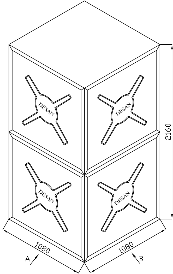
GENEL GÖRÜNÜŞÜ
