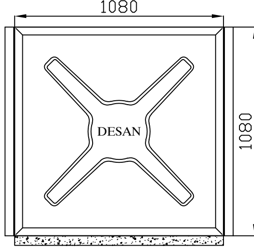
A GÖRÜNÜŞÜ
