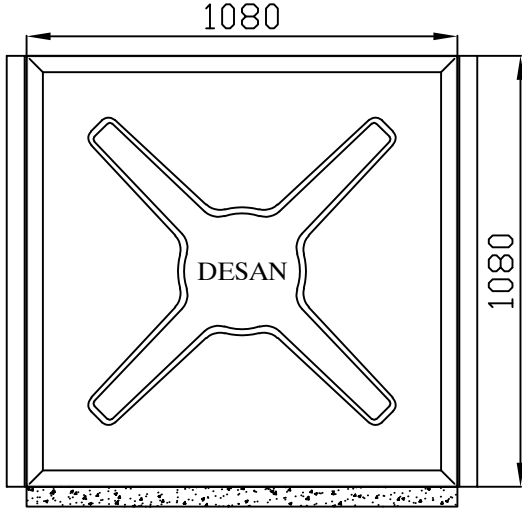
B GÖRÜNÜŞÜ
